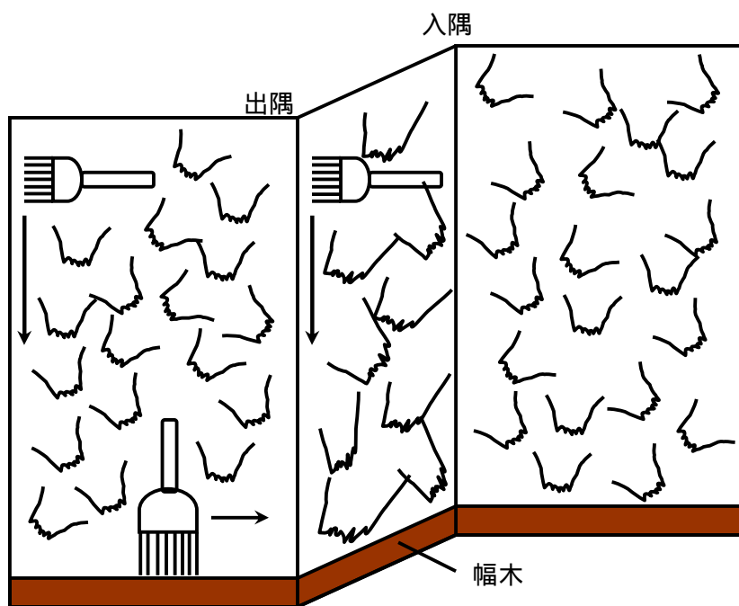
化粧目地をとる工法
