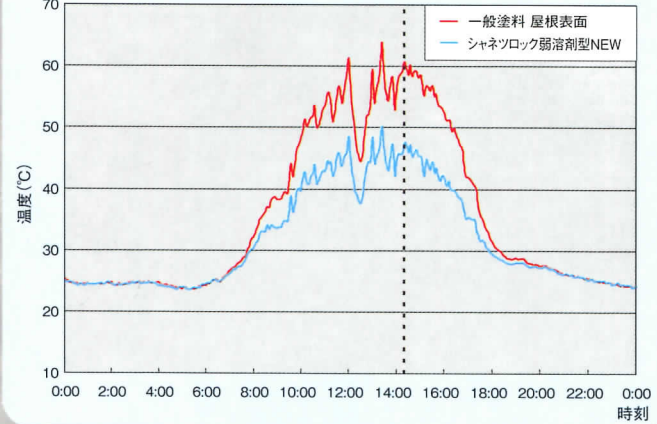
<実験棟屋根の表面温度測定結果>
