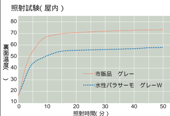
グレーを塗装した塗板を室内でランプ照射し、塗板の裏面温度を測定した結果です。
