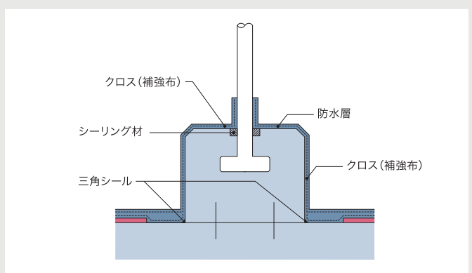
PCa板取り合い(通気緩衝工法の場合)
