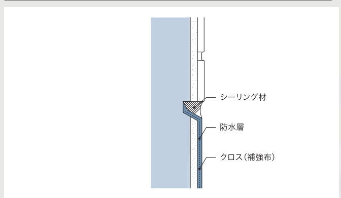
出巾木
