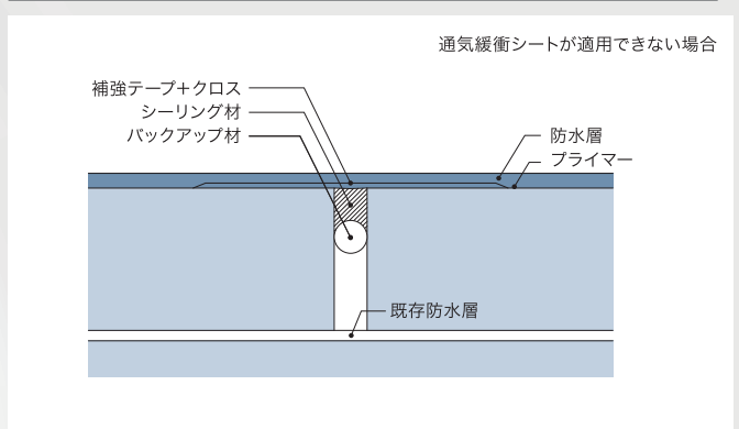
開口部
