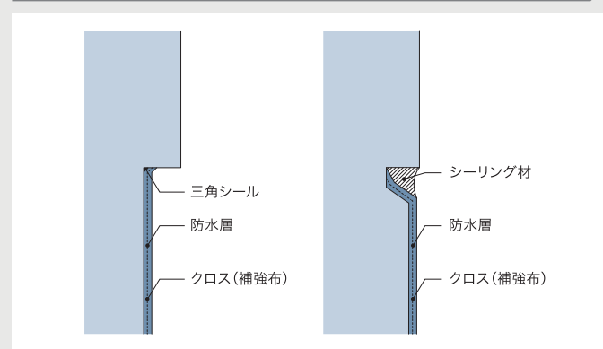
入巾木
