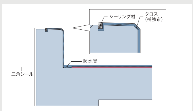
タイル壁取り合い
