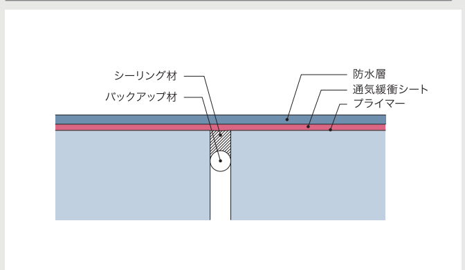
押えコンクリート伸縮目地部 (KFシールテクトWP密着工法の場合)
