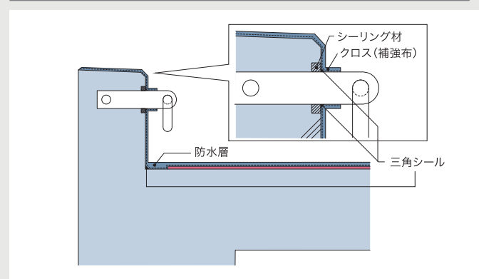
立上り 目地設置
