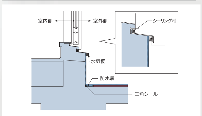
開口部
