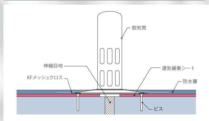
脱気筒回り
