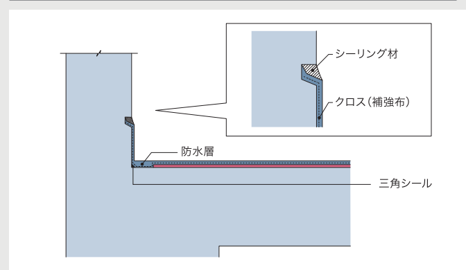
入巾木
