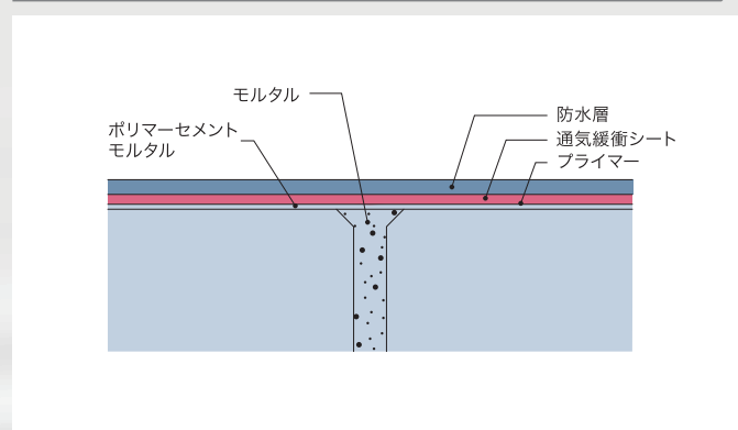
押えコンクリート伸縮目地部 (KFシールテクトWP通気緩衝工法の場合)
