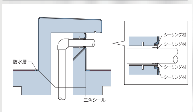
鳩小屋
