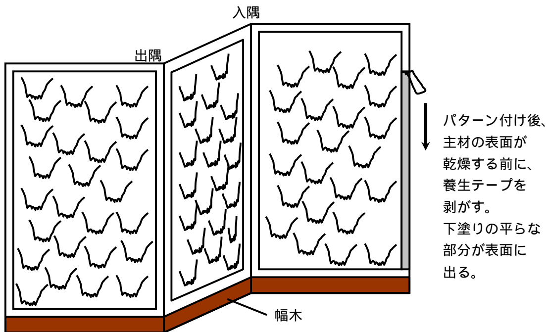
化粧目地をとる工法
