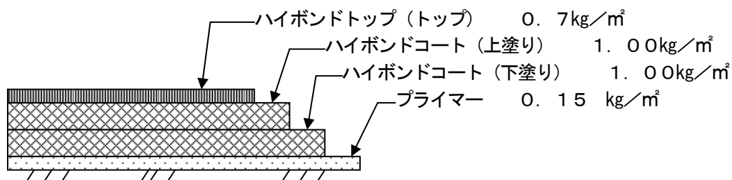
[施工図]
