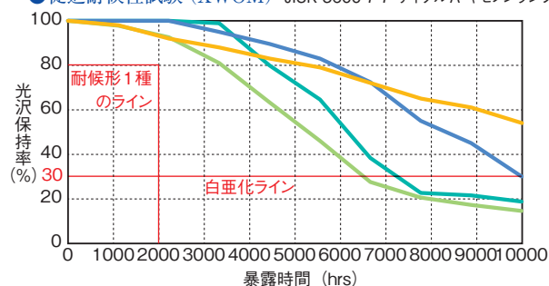
●促進耐候性試験 (XWOM) JISK 5600-7-7 サイクルA キセノンランプ法
